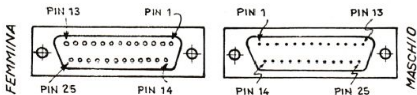
Figura 1. Connessioni nel sistema seriale standardizzato RS-232.
